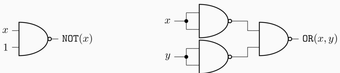
Afbeelding 3. NOT-gate (links) en OR-gate (rechts) opgebouwd uit NAND-gates. De NOT-gate heeft als invoer een bit x en een constante bit met waarde 1. Voor de OR-gate wordt de bit x gekopieerd en dubbel ingevoerd in de NAND-gate (dit is ook een manier om de NOT-gate te bouwen); hetzelfde geldt voor de bit y . De resultaten hiervan worden ingevoerd in nog een NAND. Ga vooral zelf na of al deze operaties doen wat je verwacht door een waarheidstabel te maken.
