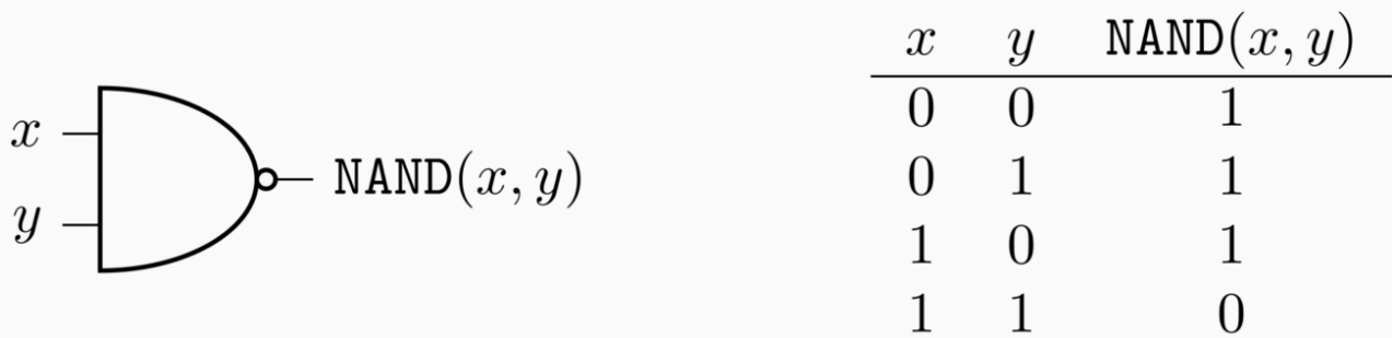
Afbeelding 2. Circuitdiagram (links) en waarheidstabel NAND (rechts). De NAND-gate heeft twee klassieke bits x en y als invoer. De werking staat rechts en is als verwacht een geïnverteerde AND-gate.
